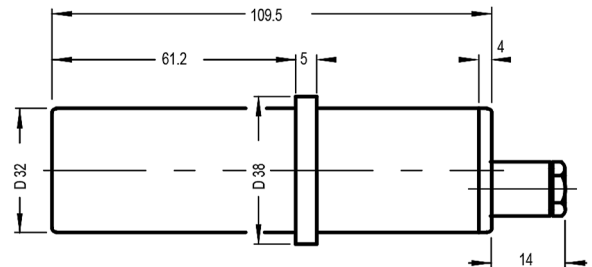
Maße (mm)
